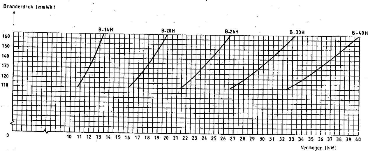
Figuur 6 : Grafiek branderdruk t.o.v. vermogen.
