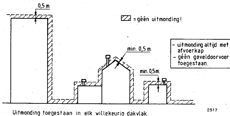
Figuur 4 : Uitmondingsgebied rookgasafvoer.
