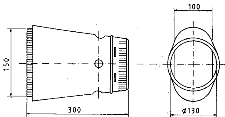
Figuur 1 : Dubbelwandig verloopstuk.
